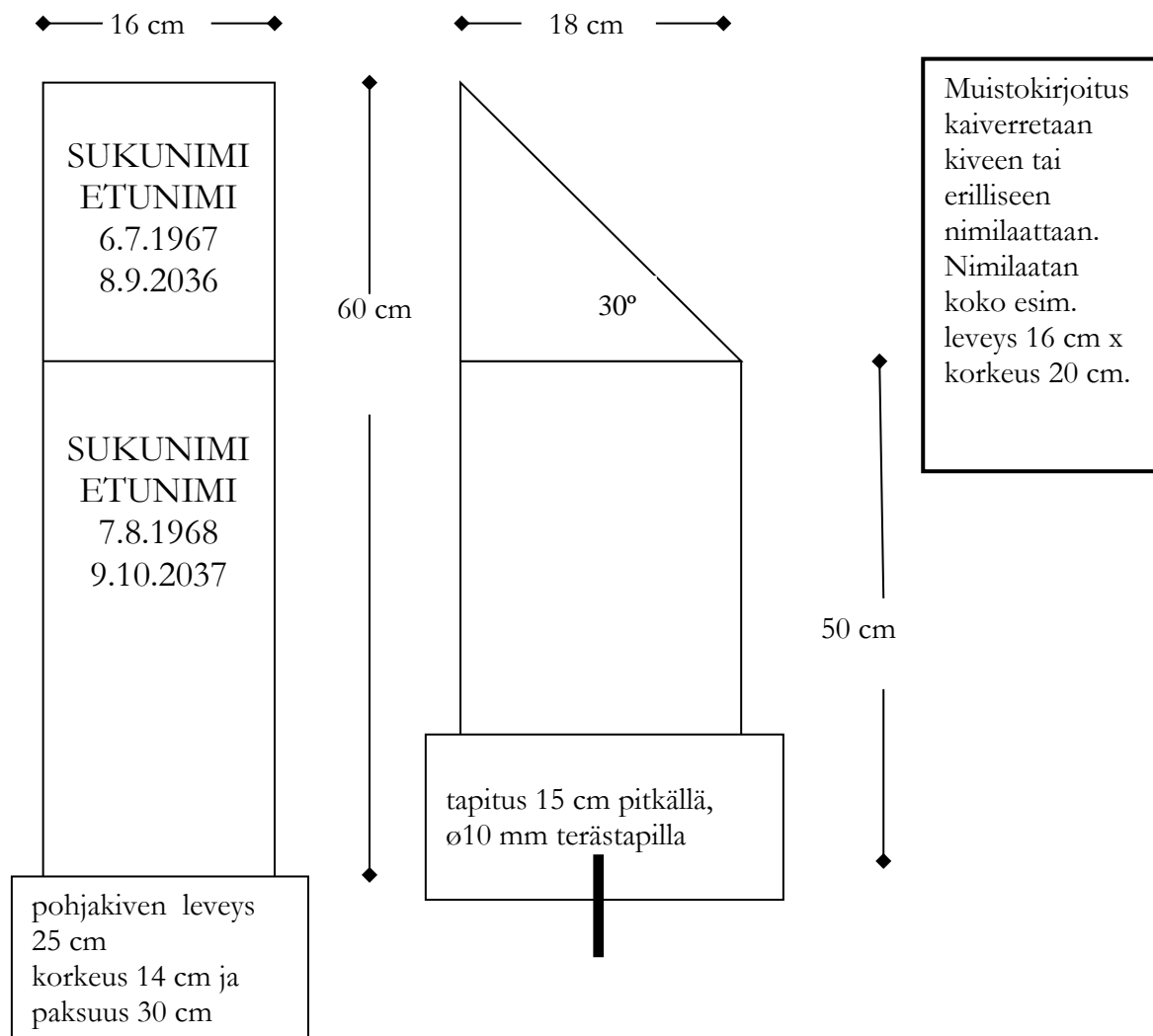
Kuva 2. P-osaston tyypikivimalli.
